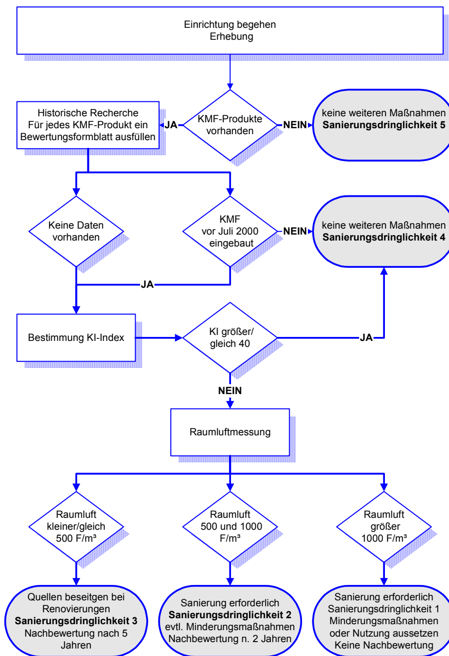
Ablaufschema Erhebung und Bewertung KMF in Gebäuden der Stadt Nürnberg
