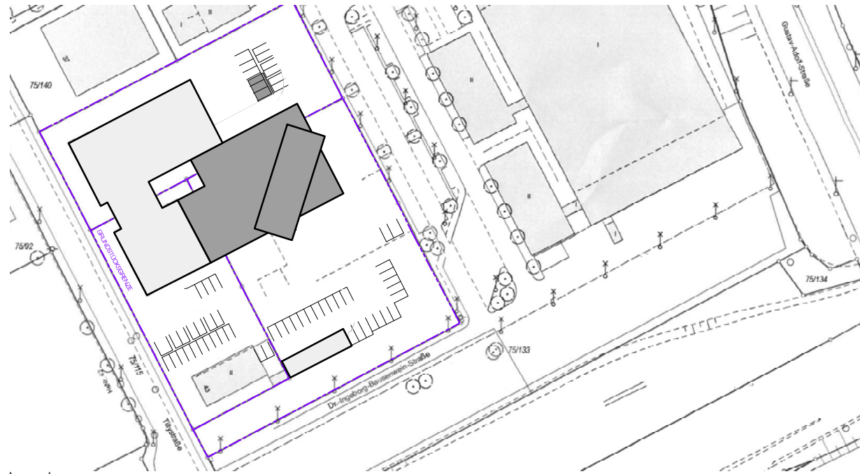
Lageplan
