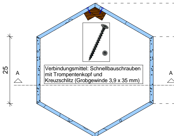
Schnitt B-B
