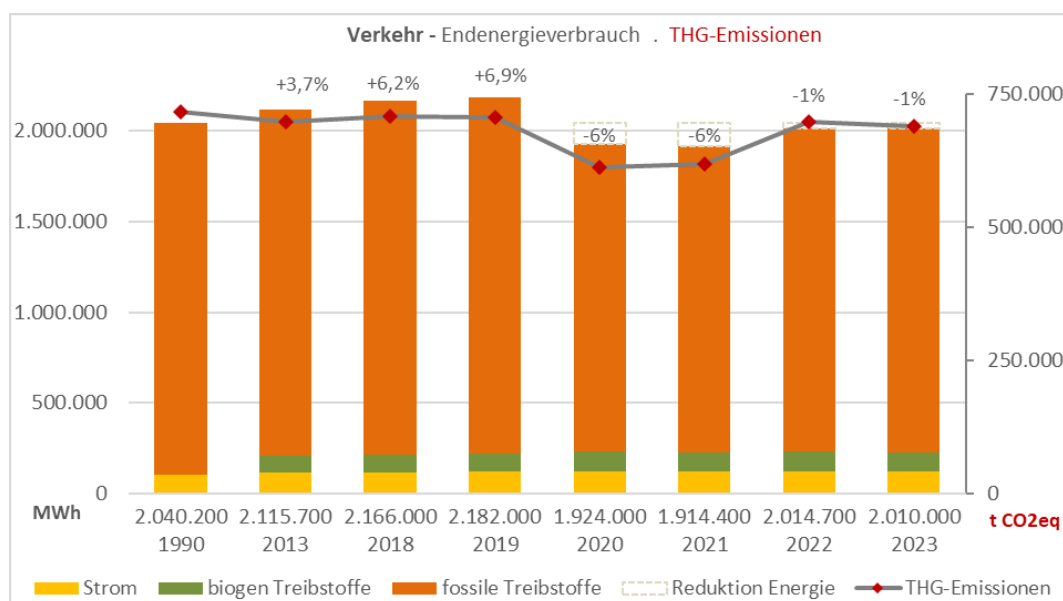
Abbildung 17: Verkehr – Endenergieverbrauch, THG-Emissionen 1990, 2013, 2018 bis 2023 2
