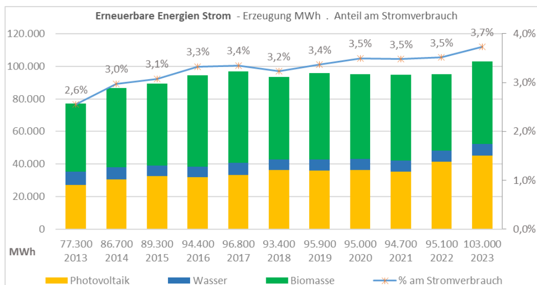
Abbildung 21: Erneuerbare Energien Strom - EEG Einspeisung 2013 bis 2023
