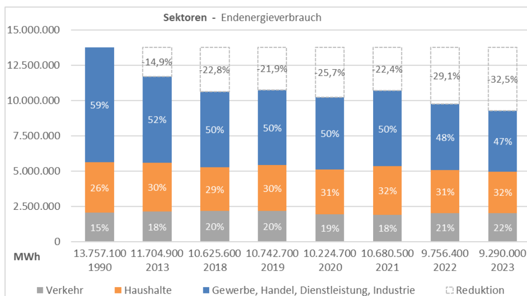
Abbildung 4: Sektoren - Endenergieverbrauch 1990, 2013, 2018 bis 2023
