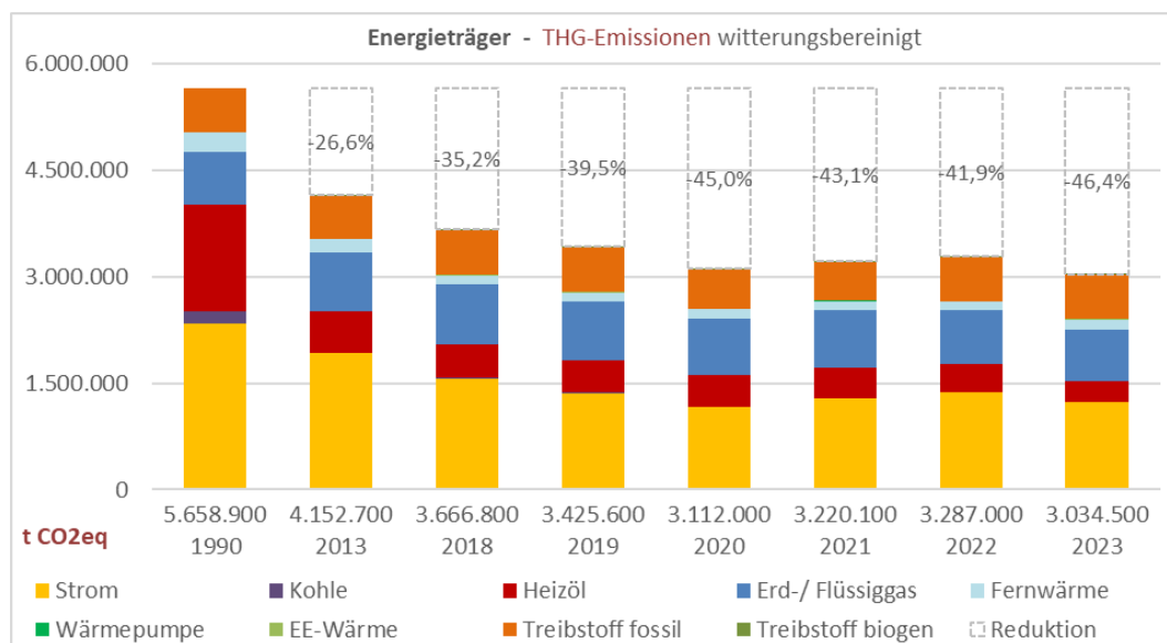
Abbildung 11: Energieträger - THG-Emissionen witterungsbereinigt 1990, 2013, 2018 bis 2023
