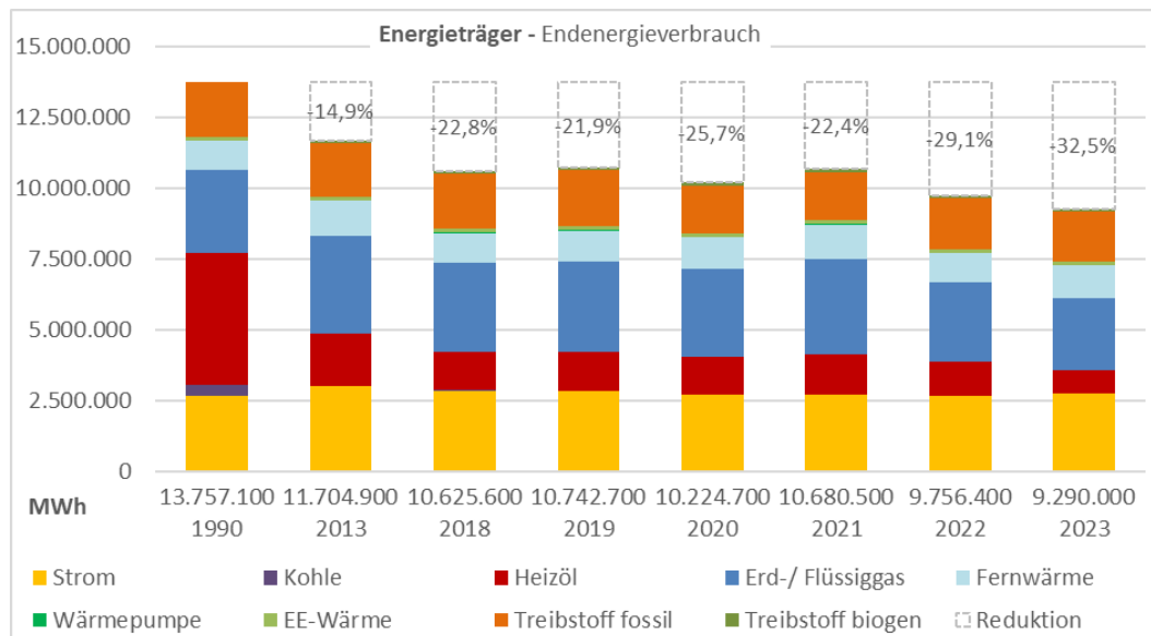
Abbildung 2: Energieträger – Endenergieverbrauch 1990, 2013, 2018 bis 2023
