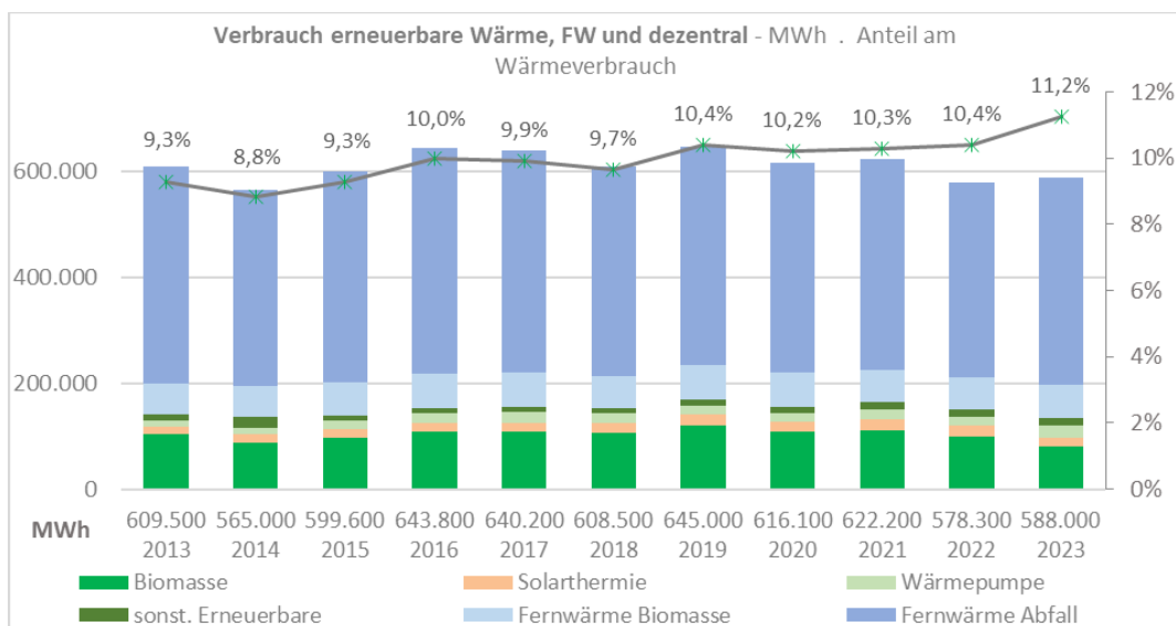
Abbildung 20: Verbrauch erneuerbare Wärme, Fernwärme und dezentral, 2013 bis 2023
