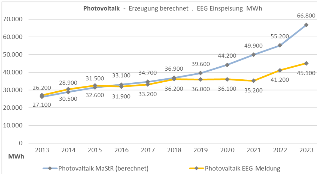
Abbildung 23: Photovoltaik – Erzeugung berechnet. EEG Einspeisung
