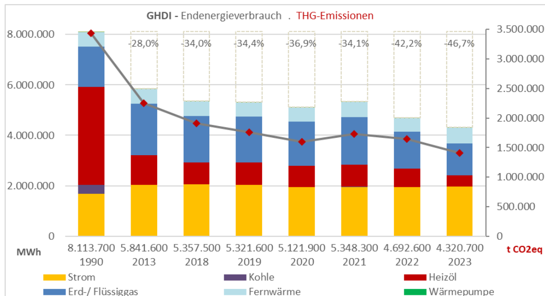
Abbildung 13: GHD – Endenergieverbrauch, THG-Emissionen 1990, 2013, 2018 bis 2023
