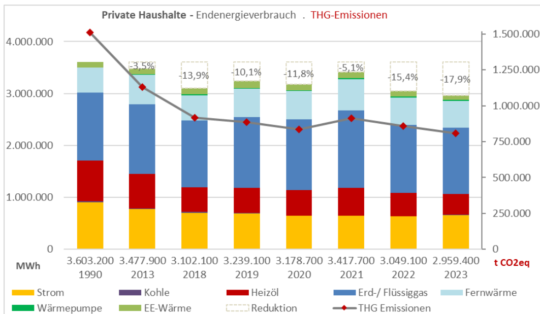
Abbildung 15: Private Haushalte – Endenergieverbrauch, THG-Emissionen 1990, 2013, 2018 bis 2023
