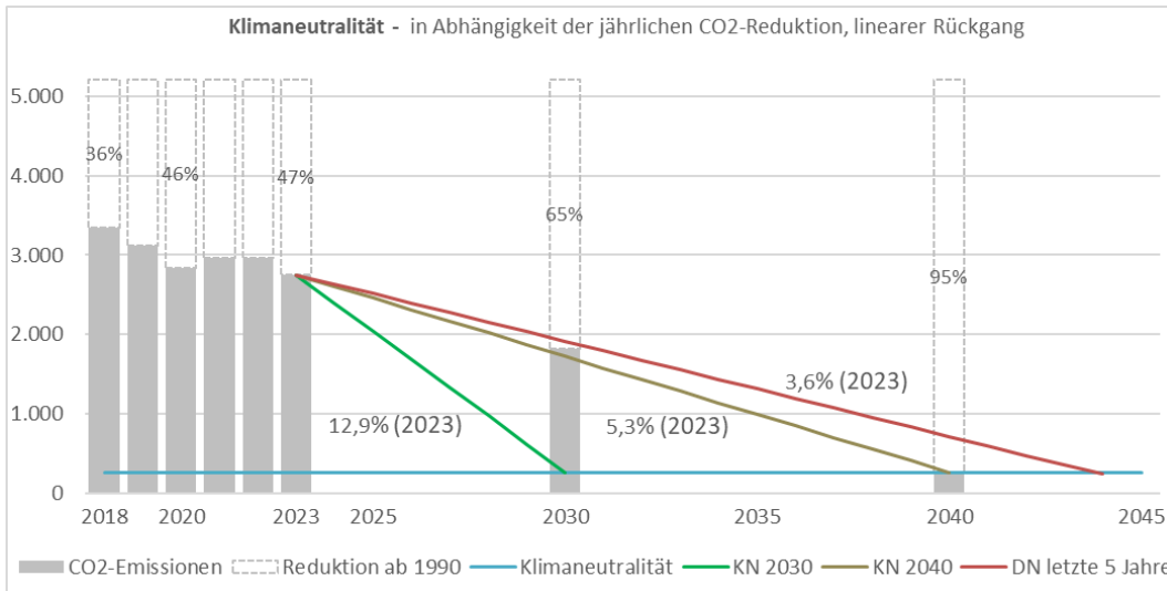
Abbildung 25: Klimaneutralität, in Abhängigkeit der jährlichen CO 2 -Reduktion, linearer Rückgang
