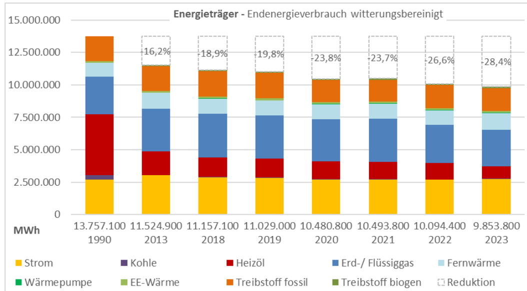
Abbildung 10: Energieträger – Endenergieverbrauch witterungsbereinigt 1990, 2013, 2018 bis 2023
