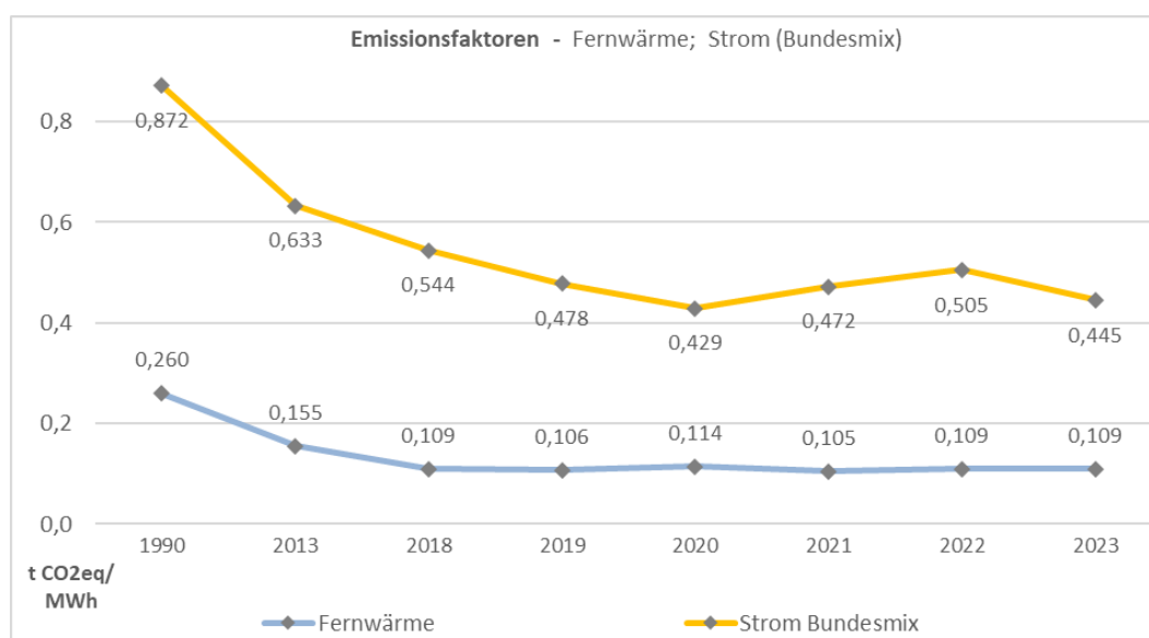
Abbildung 8: Emissionsfaktor Strom und Fernwärme 1990, 2013, 2018 bis 2023
