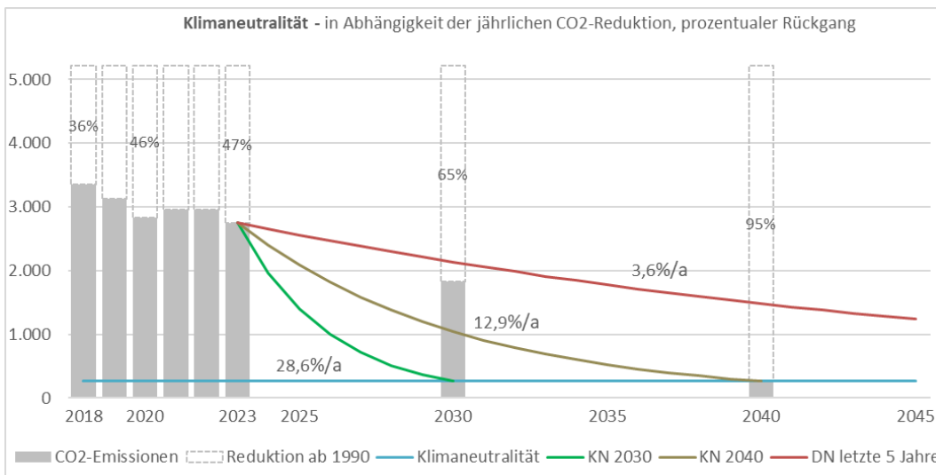
Abbildung 26: Klimaneutralität, in Abhängigkeit der jährlichen CO 2 -Reduktion, prozentualer Rückgang
