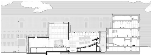
Schnitt durch Bestand und Ergänzungsbau
