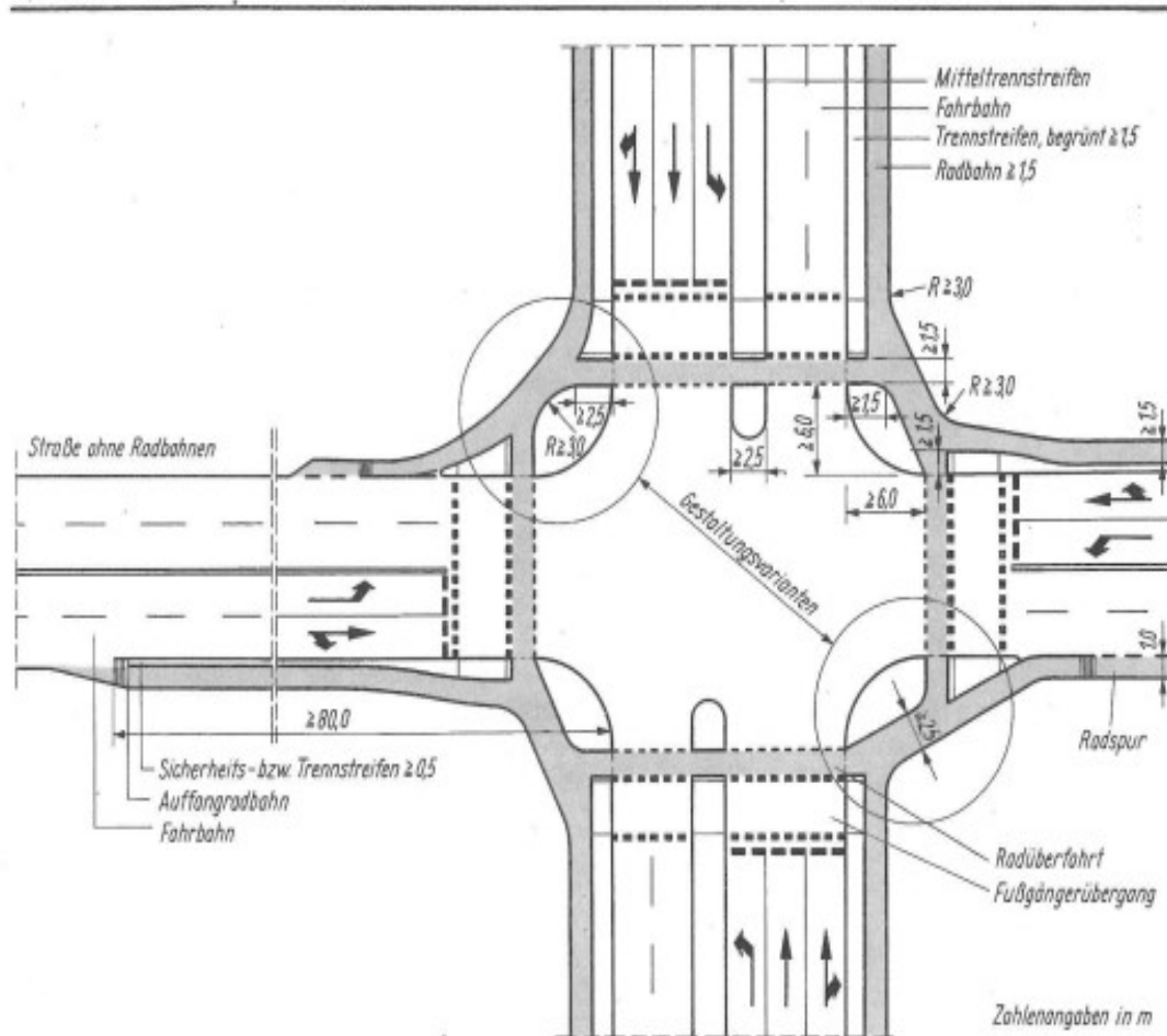
Bild 3-33. Führung des Radverkehrs an Straßenknoten mit dem Fußgängerverkehr (starre Schiene)
