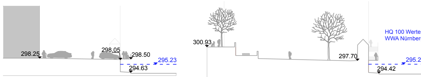
SCHNITT A-A'
