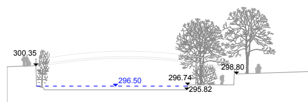
SCHNITT A-A
