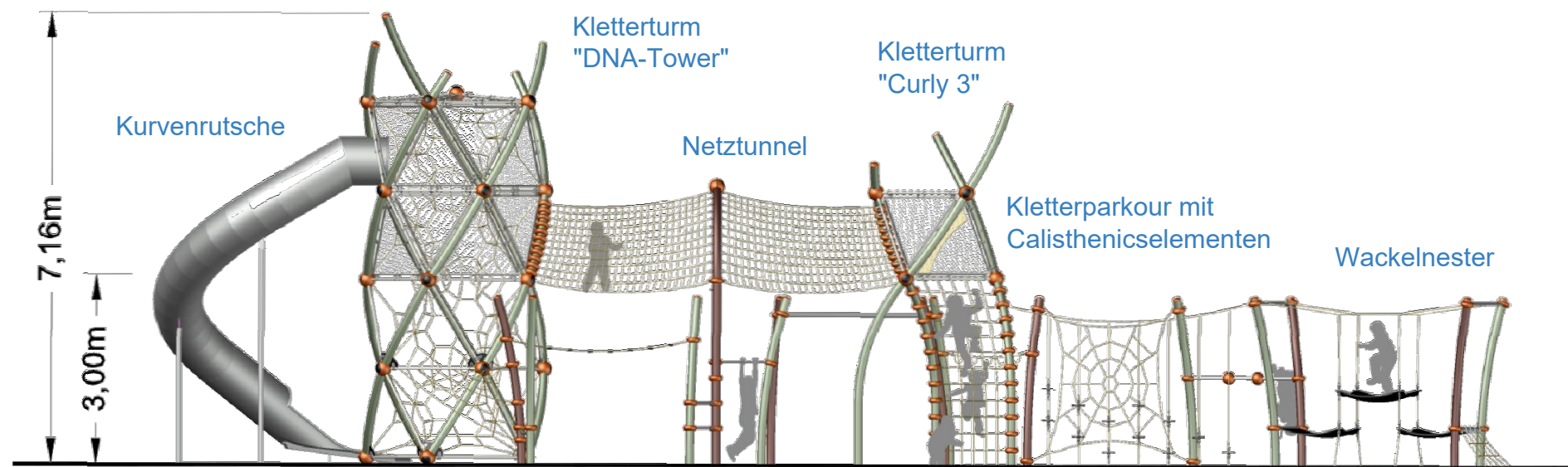
Spielgerät - Seitenansicht M: 1:100
