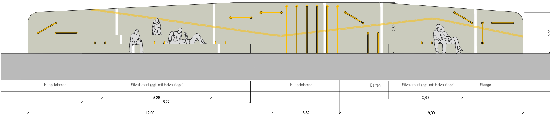
Abwicklung Spielmauer mit Sitz- und Fitnessselementen
