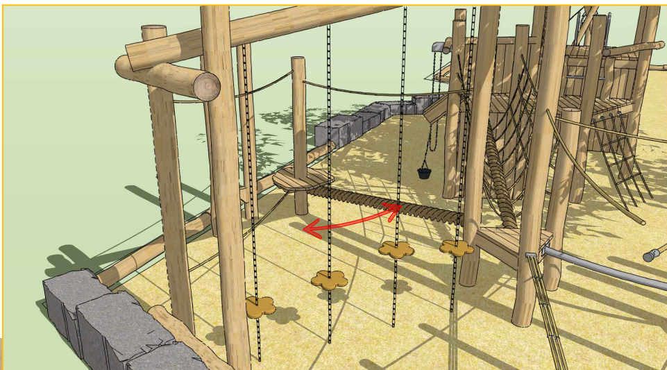
8 Tritttelleranlage
