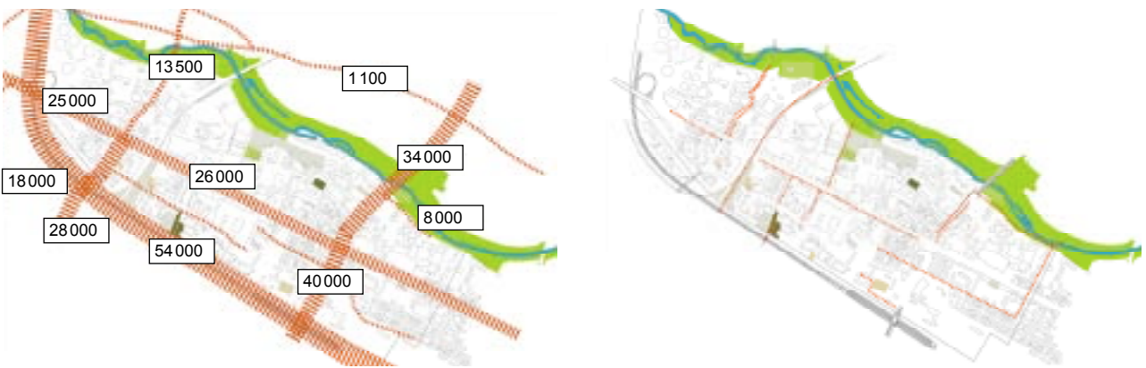
■ 10 Tägliches Kfz-Aufkommen auf den Straßen in der Nürnberger Weststadt und Umgebung (eigene Darstellung nach [Nürnberg 2012], [Verkehr Nürnberg 2012]) ■ 11 Fehlende Radwege(-verbindungen) in der Nürnberger Weststadt (eigene Darstellung nach [Alam 2012])
