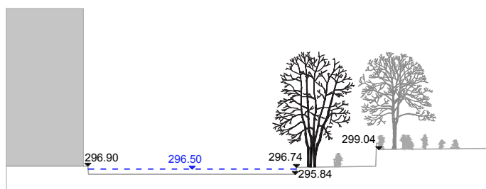
SCHNITT B-B'
