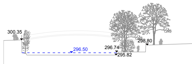
SCHNITT A-A'
