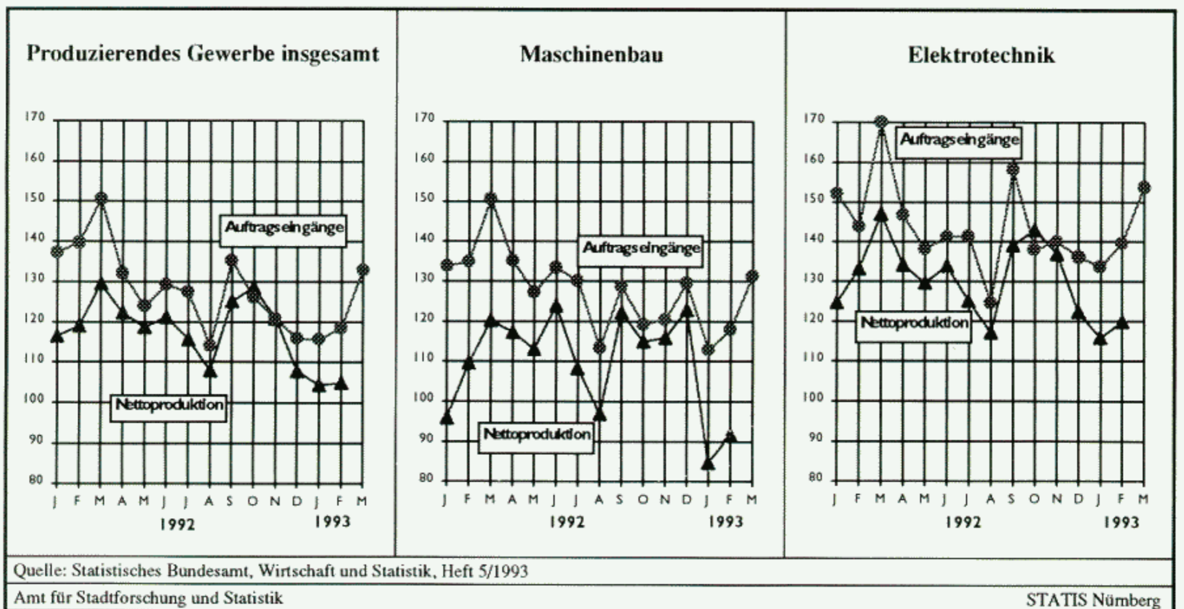
Abb. 4: Index der Nettoproduktion (arbeitstäglich bereinigt) und Index der Auftragsengänge des Produzierenden Gewerbes insgesamt, des Maschinenbaus und der Elektrotechnik im Bundesgebiet (alte Länder) von Januar 1992 bis März 1993 (Index 1985 = 100)
