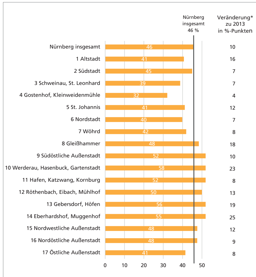
Abb. 11: Ist Ihrer Meinung nach die Polizei ausreichend gegenwärtig? (Antwortanteil „nein“ nach Umfragegebieten, in Prozent)
