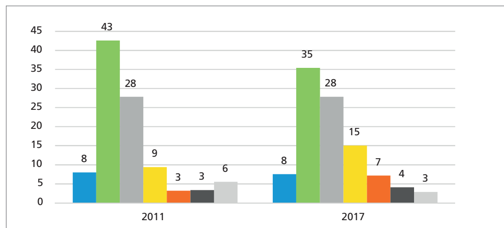
Abb. 1: Zufriedenheit mit öffentlicher Sicherheit, Schutz vor Kriminalität* 2011 und 2017, in Prozent
