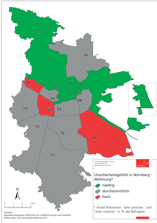
Karte 1: Unsicherheitsgefühl in Nürnberg - Wohnung nachts (Umfragegebiete)
