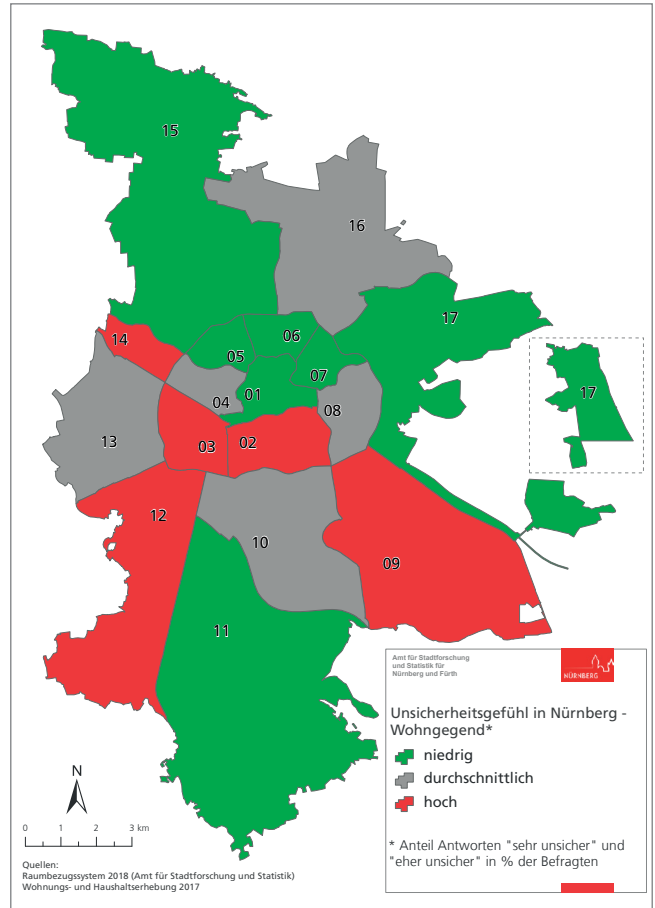
Karte 2: Unsicherheitsgefühl in Nürnberg - Wohngegend nachts (Umfragegebiete)
