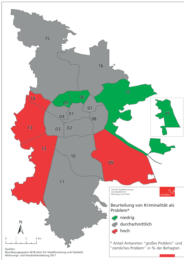
Karte 3: Beurteilung von Kriminalität als Problem (Umfragegebiete)
