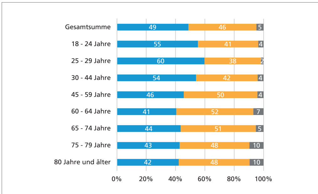
Abb. 10: Ist Ihrer Meinung nach die Polizei ausreichend gegenwärtig? (nach Altersgruppen, in Prozent)
