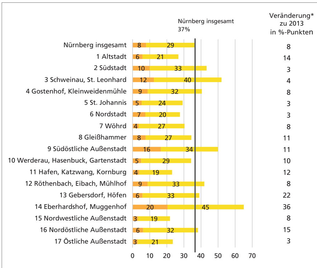
Abb. 6: Sicherheitsgefühl in der Wohngegend nachts nach Umfragegebieten, Antwortanteile „sehr unsicher“ und „eher unsicher“, in Prozent
