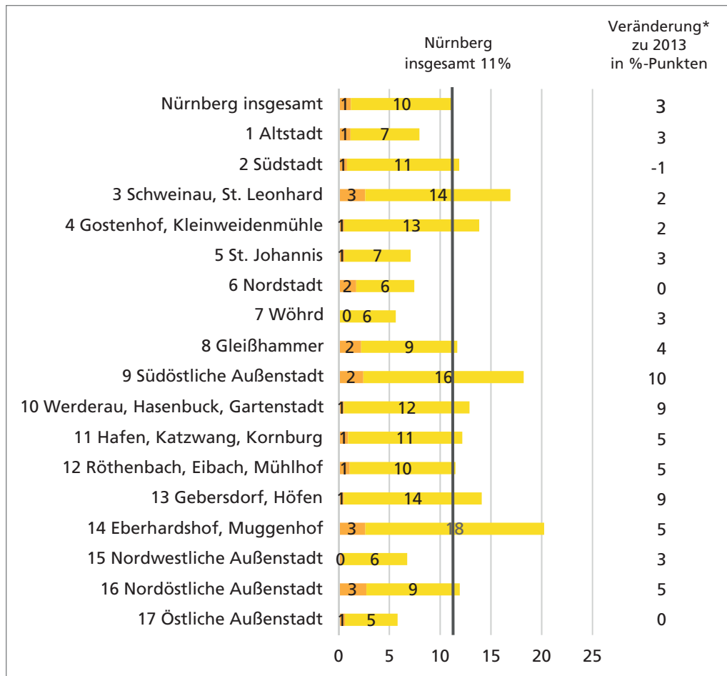
Abb. 4: Sicherheitsgefühl in der Wohnung nachts nach Umfragegebieten, Antwortanteile „sehr unsicher“ und „eher unsicher“, in Prozent
