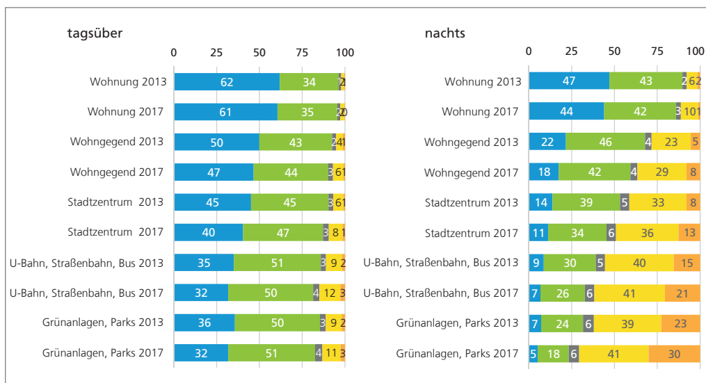
Abb. 2: Sicherheitsgefühl* in Nürnberg 2013 und 2017, in Prozent
