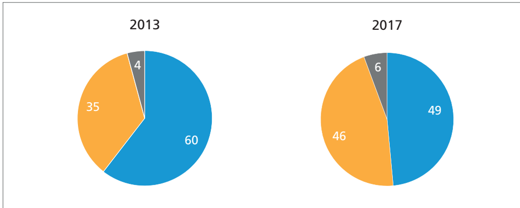
Abb. 9: Ist Ihrer Meinung nach die Polizei ausreichend gegenwärtig? (in Prozent)
