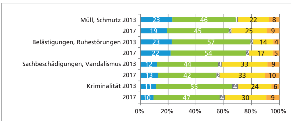
Abb. 7: Beurteilung von Sicherheit und Ordnung* in Nürnberg 2013 und 2017, in Prozent
