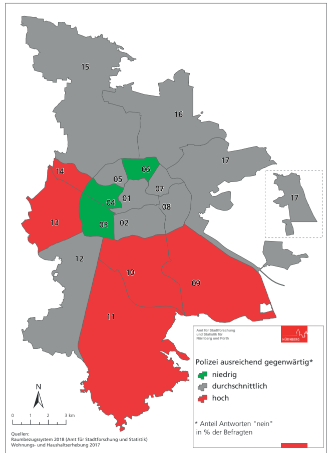
Karte 4: Polizei ausreichend gegenwärtig (Umfragegebiete)
