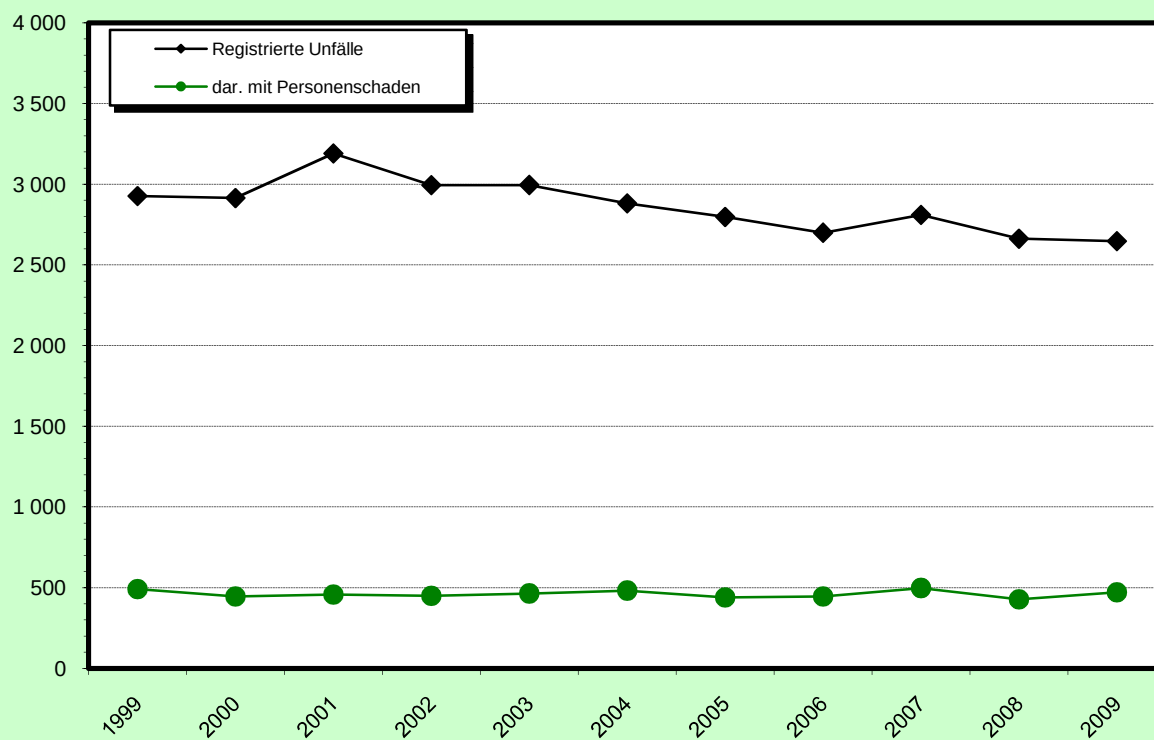
Schaubild: Straßenverkehrsunfälle
