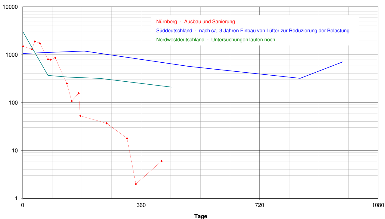
Vergleich der 2-Chlorpropan-Konzentration in der Raumluft von Kindertagesstätten nach Einbau von Phenolharz-Hartschaumplatten im Bodenaufbau
