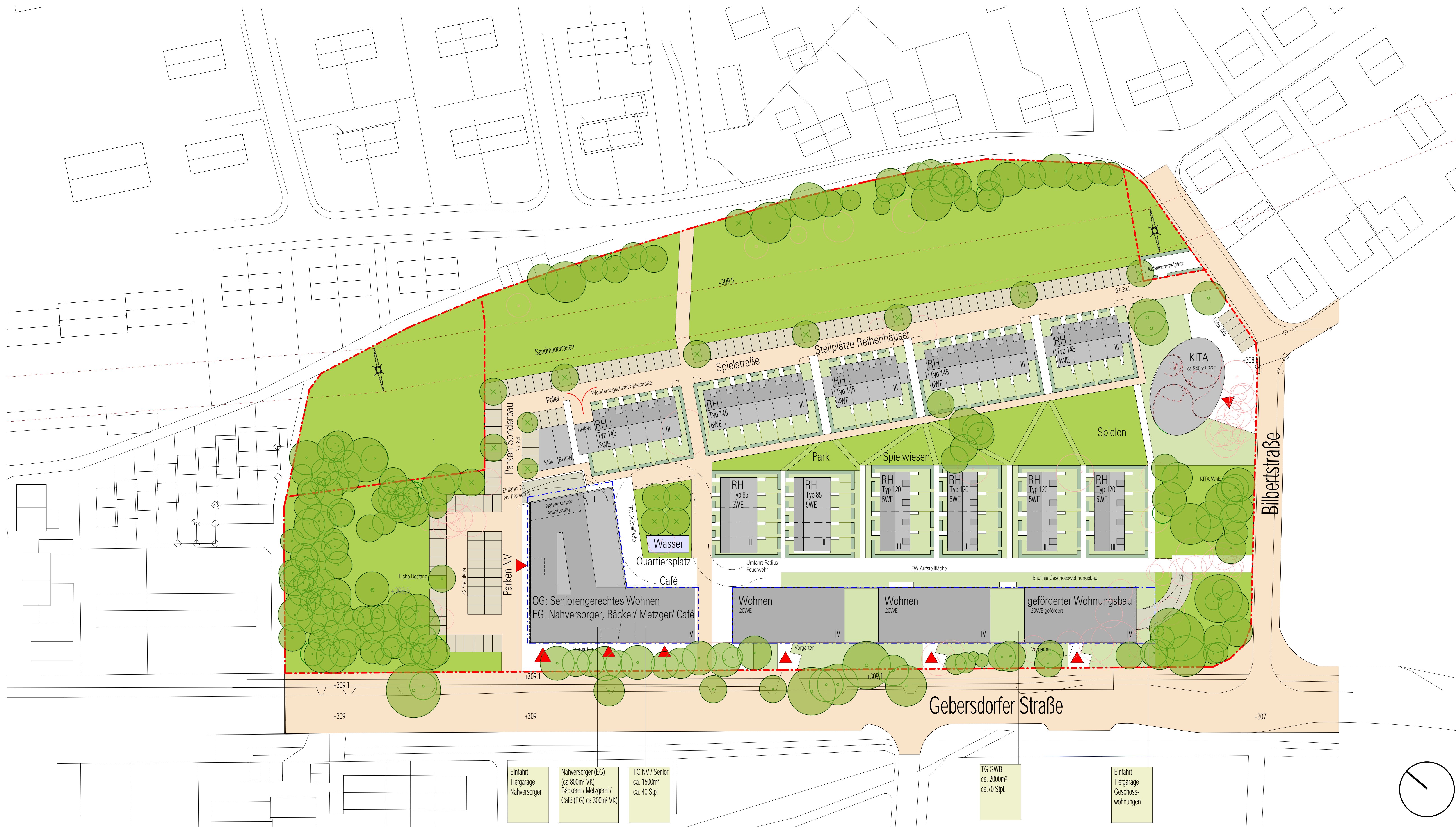
Lageplan M 1:500
